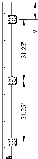
HINGE JAMB
